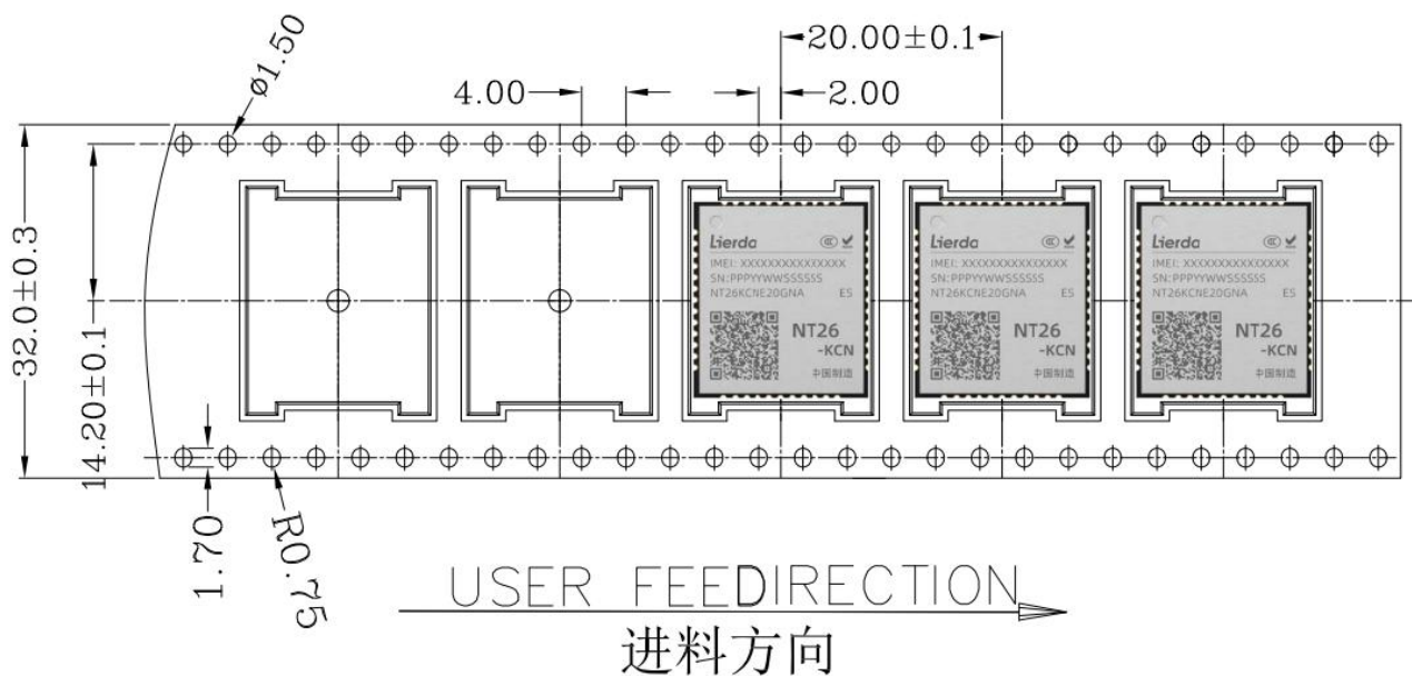
图 9-3 载带进料方向指示图
