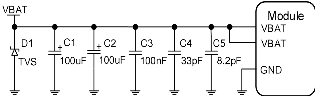
图 3-4 模组供电电路参考
